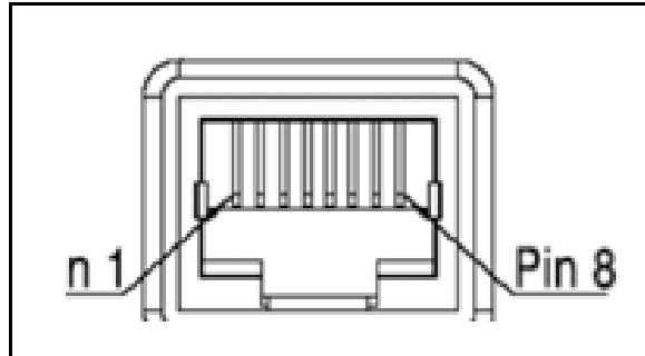
Şekil 5 – E1 G.703 RJ45 (dişi) konnektör (Pin 1 ... Pin 8)
